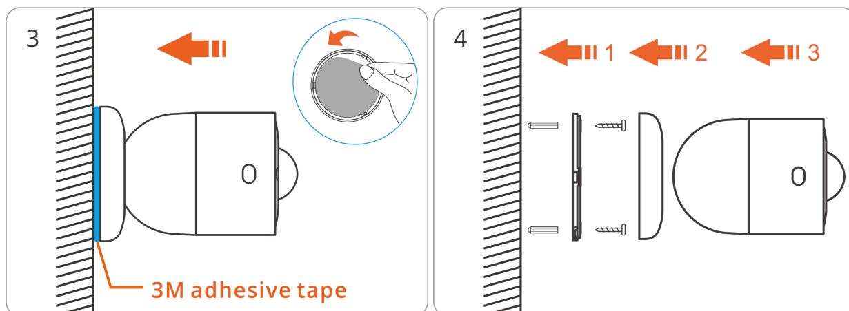
3) Přilepení na stěnu oboustrannou lepicí páskou 3M na podstavci. 4) Přišroubování podstavce na stěnu.
