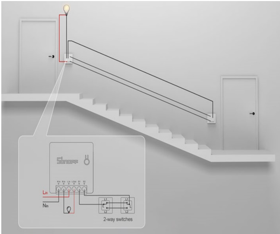
Schéma schodišťového zapojení:
