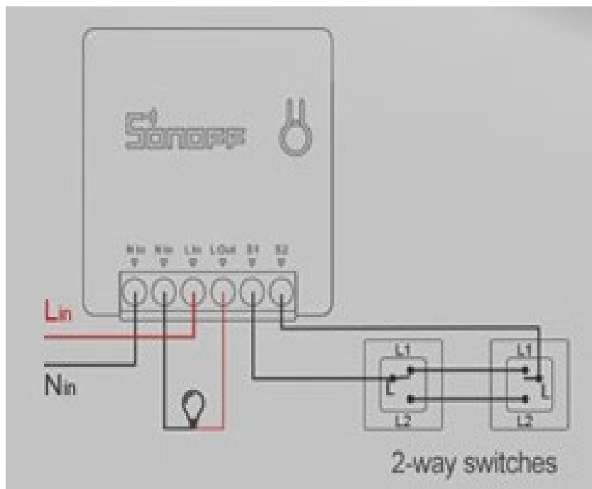
Schéma schodišťového zapojení:
